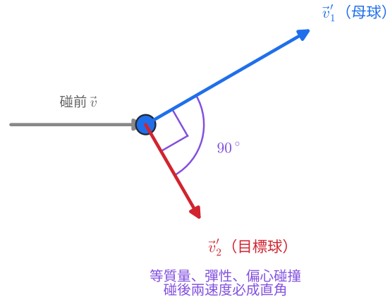
圖 1-3：二維碰撞。左——動量向量守恆：碰前總動量 \vec{p} 等於碰後兩動量 \vec{p}_1' 、 \vec{p}_2' 的向量和（平行四邊形法則）；拆成分量看， x 分量相加守恆、 y 分量上下抵消（碰前 y 分量為零）。右——一動一靜、等質量的兩球作彈性偏心碰撞，碰後兩速度 \vec{v}_1' 、 \vec{v}_2' 必互相垂直（夾 90^\circ ），即撞球的直角分開現象。
