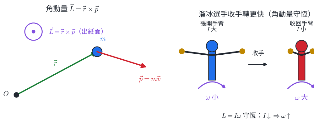
圖 1-5：左——角動量 \vec{L} = \vec{r} \times \vec{p} ，大小為 rp \sin \theta ，方向由右手定則決定 (此例出紙面)。右——溜冰選手收手：質量靠近轉軸使轉動慣量 I 變小，由 L = I\omega 守恆，角速度 \omega 隨之變大。
